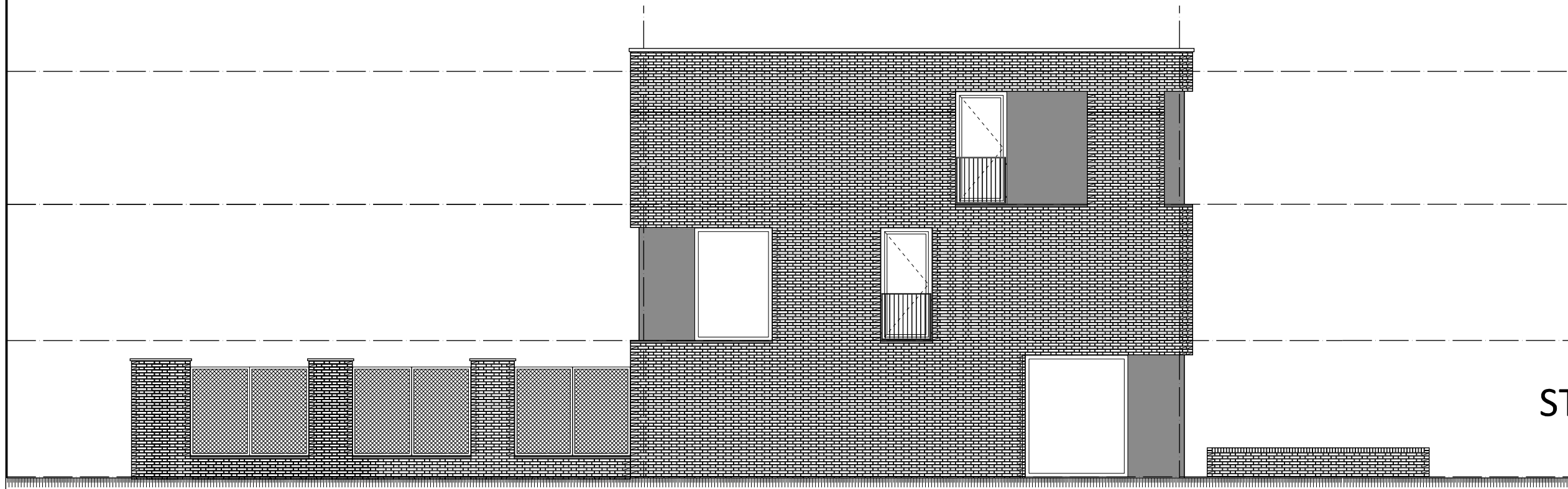
ACHTERGEVEL
